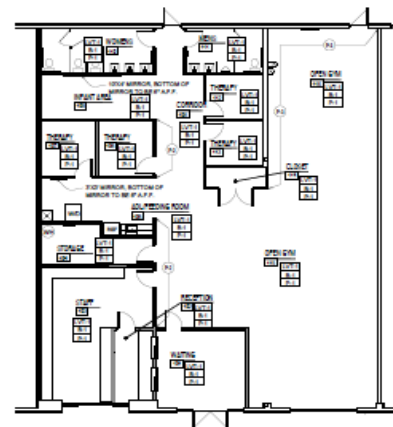
1 FINISH PLAN SCALE: 1/8" = 1'-0"
